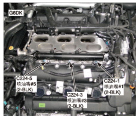
48. 发动机右侧
