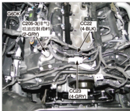
44. 发动机前部
