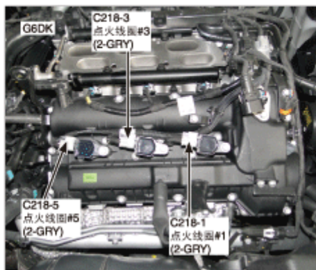
47. 发动机右侧
